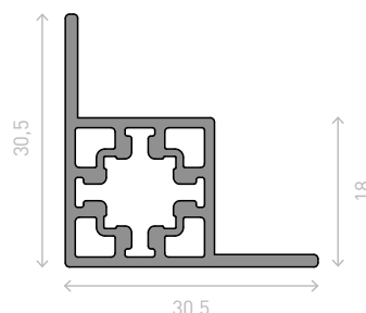
Doppel-Seiten-/Bodenprofil 83326
