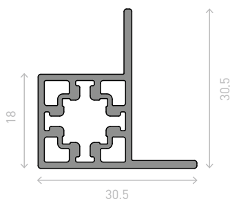
Doppel-Seiten-/Bodenprofil 83325
