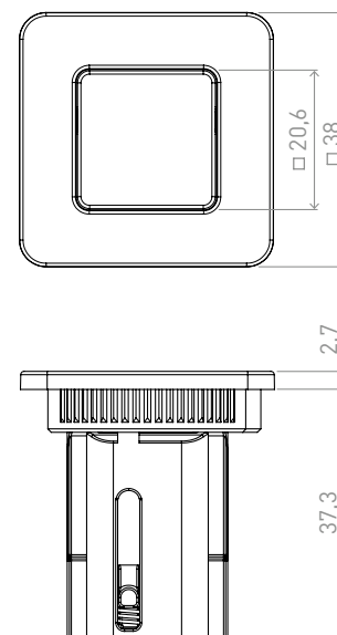
Bouton fonctionnel
