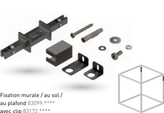
1 Fixation murale / au sol 83096.*** 2 Fixation murale / au sol 83147.***
