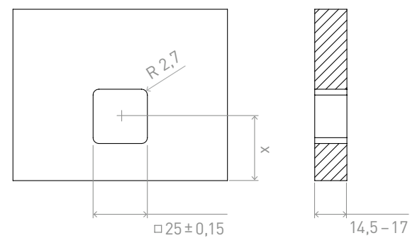
Schéma de fraisage
